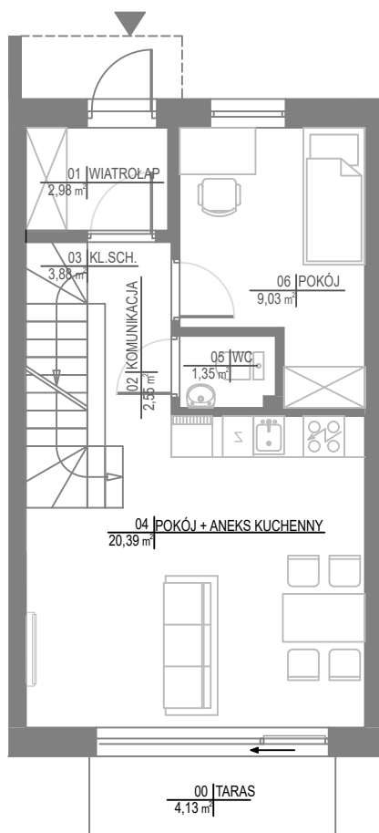
RZUT PARTERU
